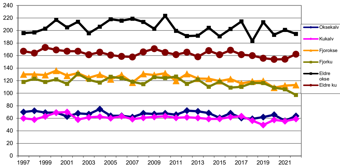
Figur 3: Gjennomsnittvekter på elg, hhv oksekalv, kukalv, fjorokse, fjorku, eldre okse og eldre ku, for statsallmenningen i Engerdal perioden 1997 – 2022.
