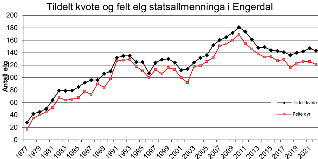
Figur 1: Tildelt kvote og felt elg på statsallmenninga for perioden 1977-2022.
